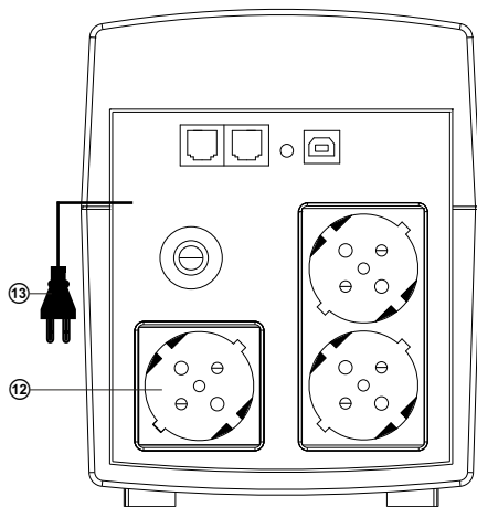
Задняя панель ИБП Pro 1000 (USB)/Pro1500 (LCD, USB)
