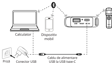
Fig. 5. Schema de conectare
