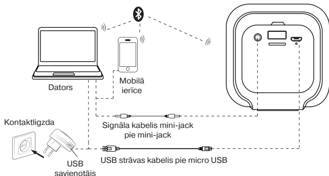
2. att. Pieslēgšanas shēma
