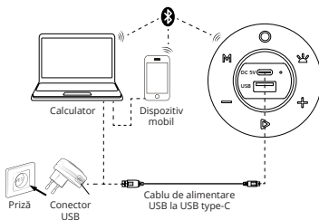
Fig. 2. Schema de conectare
