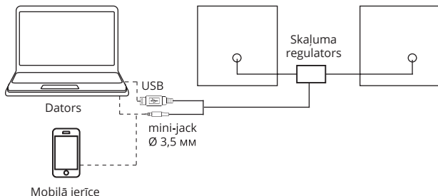
1. att. Pieslēgšanas shēma
