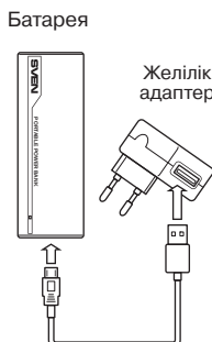
3-сур. Батареяның желілік адаптерден зарядталуы
